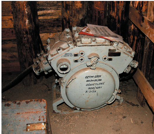
Ryc. 3. Ognioszczelny wyłącznik typu KWSOI 160-24
