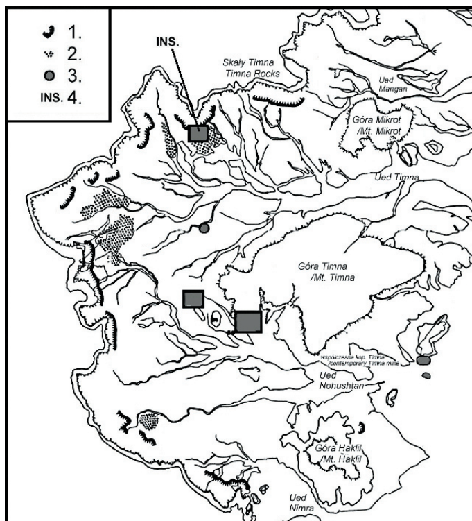
Ryc. 3. Mapa kopalń w Timna (Izrael) (wg Wimmera, 2010); 1. starożytne kopalnie, 2. doły po płukaniu urobku, 3. miejsca prowadzenia wykopalisk, 4. miejsce odnalezienia inskrypcji
